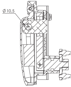
KESİT A-A
