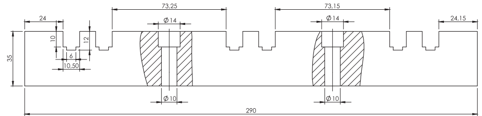
Tarak İzolatör 3x2F / Insulator 3x2F
