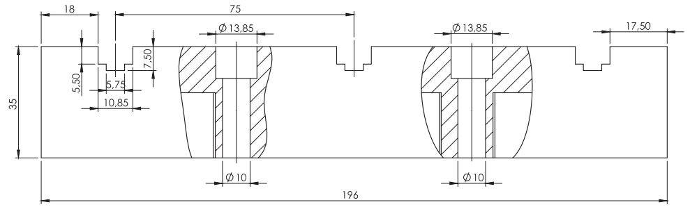
Tarak İzolatör 3x1F / Insulator 3x1F
